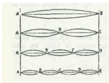
Fig. 77. — Resonancia simultánea de las partes alícuotas de una cuerda vibrante.
